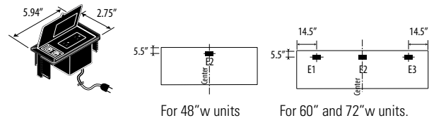
Power Block PMSPDM, Add $330 Specify location E1, E2 or E3, Add $96
