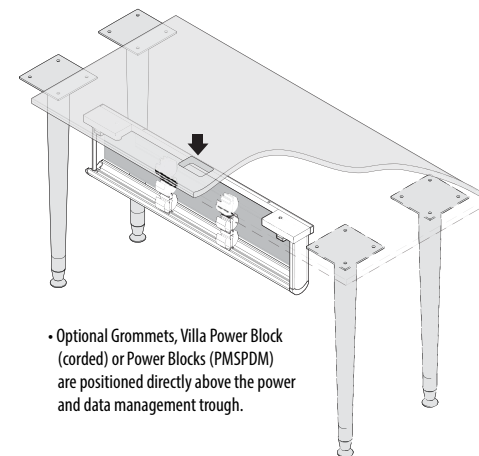
Grommet
