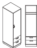
Penderie étroite
