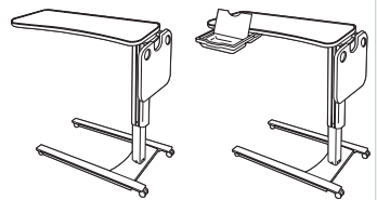
Dessus réniforme en thermoplastique, bord anti-éclaboussure, dessus rabattable, piétement en U - DROITE
