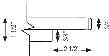
Edge Detail Foundations Casegoods
