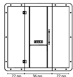
Dimensions intérieures - Vue de face
