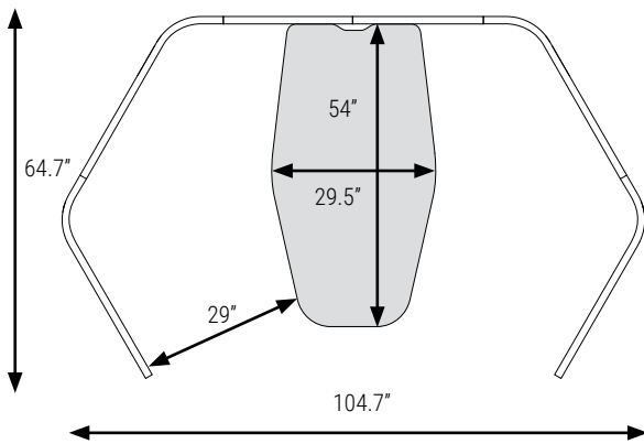
HX6PFD Alcôve Softpod avec 6 cloisons et surface en D
