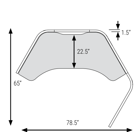
HX4P5472SW Alcôve Softpod simple avec 4 cloisons
