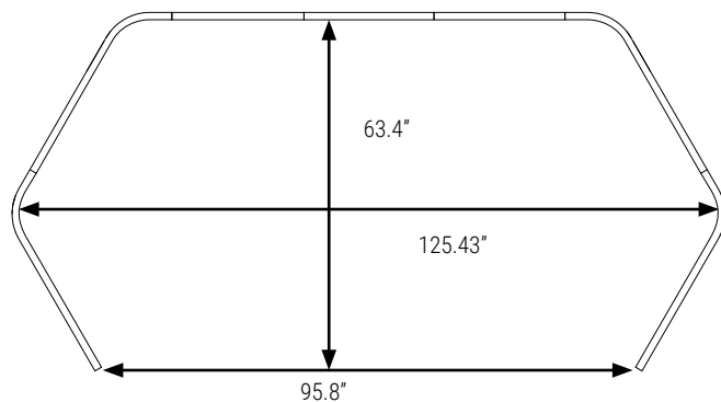
HX7PFD Alcôve Softpod avec 7 cloisons et surface en D
