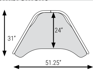
HX2P5452SW Alcôve Softpod simple avec 2 cloisons
