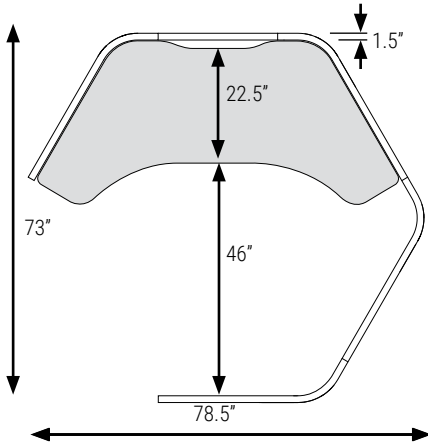
HX5P5472SW Alcôve Softpod simple avec 5 cloisons
