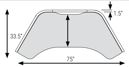
HX3PH5472SW Alcôve Softpod avec 3 cloisons et surface de travail réglable en hauteur
