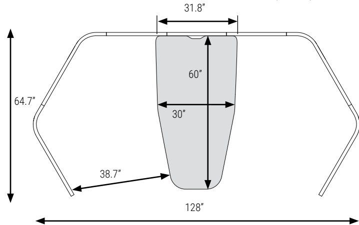
HX7PFD Alcôve Softpod avec 7 cloisons et surface en D
