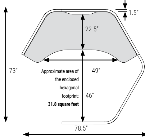
Alcôve Softpod simple avec 5 cloisons
