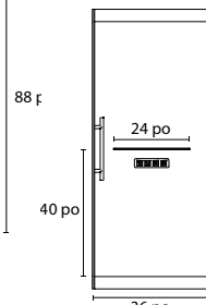
Dimensions intérieures - Vue latérale
