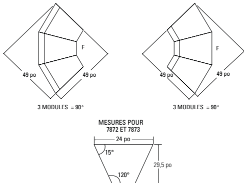
modèle 7871
