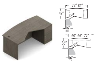
Bureau allongé à dessus arqué à un caisson - DROITE
