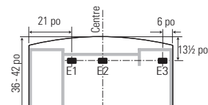
Bureau à devant arqué
