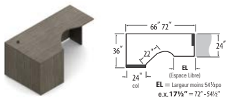
Module de coin allongé, col de 24 po - GAUCHE
