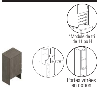
Bibliothèque de table avec porte et cavité - 43,2 po H - GAUCHE*
