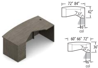
Bureau allongé à dessus arqué à un caisson - GAUCHE
