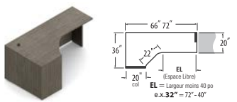
Module de coin allongé, col de 20 po - GAUCHE
