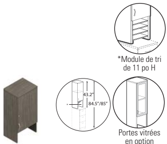
Bibliothèque de table avec porte et cavité - 43,2 po H - DROITE*
