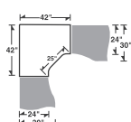
Module de coin à cinq faces, col de 24 po
