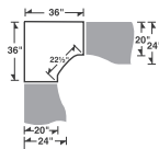
Module de coin à cinq faces, col de 20 po
