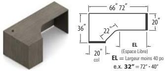
Module de coin allongé autoportant, col de 20 po - GAUCHE
