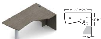
Îlot de coin allongé Panneau latéral pleine profondeur et pied (piètement en T) - GAUCHE
