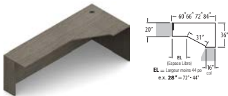
Module de coin allongé, col de 16 po - DROITE
