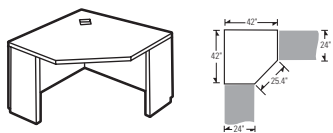
Module de coin à cinq faces
