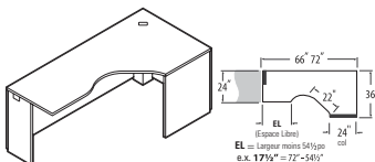
Module de coin allongé, col de 24 po - DROITE
