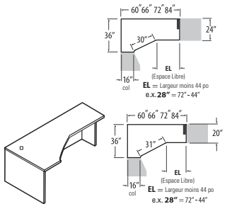
Module de coin allongé, col de 16 po - GAUCHE
