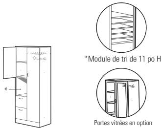
Rangement personnel avec portes et cavité - GAUCHE
