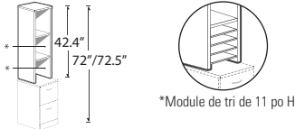
Bibliothèque de table 42,4 po H
