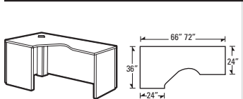
Module de coin allongé de gauche - module autoportant
