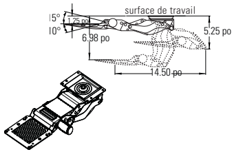
Mécanisme de tablette à clavier sans coulisses
