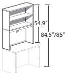
Étagère ouverte avec dos 54,9 po H
