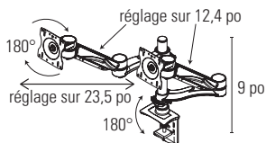
Support avec deux bras à double extension à hauteur réglable
