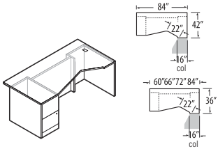
Bureau allongé à un caisson - GAUCHE
