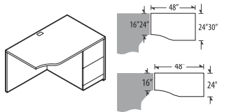
Space Saver Return - RIGHT*
