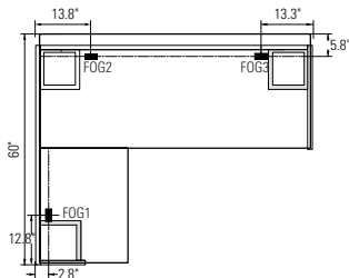
L HA desk
